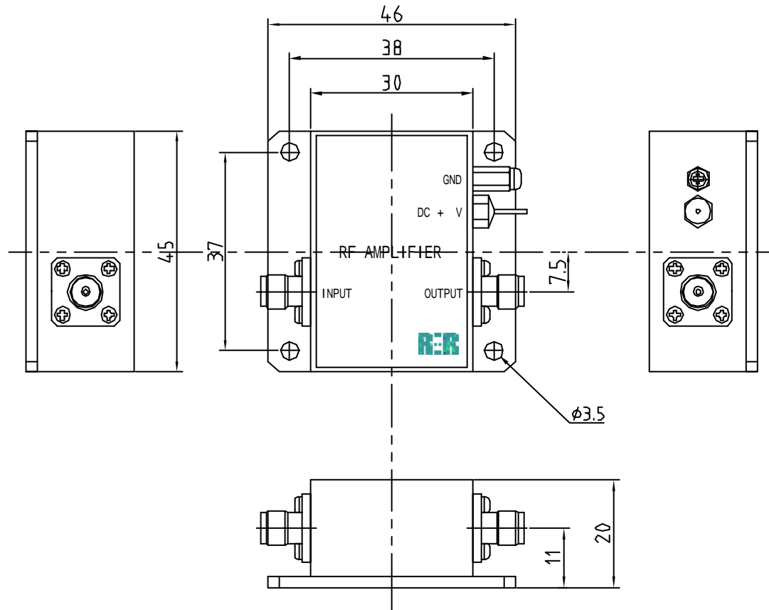
外観図 1
