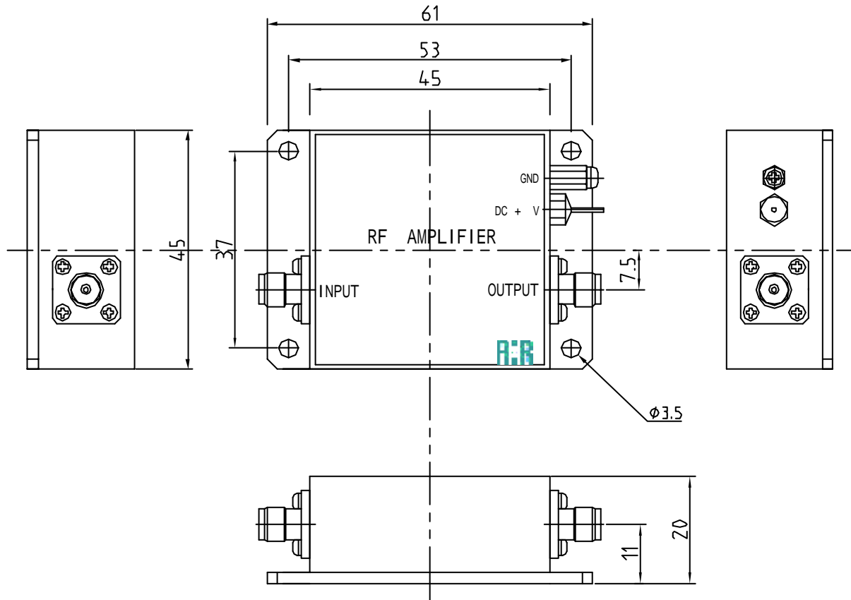
外観図 2
